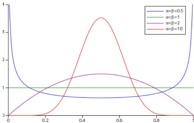
赤玉の確率 P(A) = \psi
