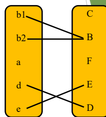
部分写像
