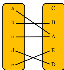
写像 (関数)
